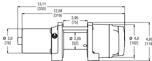
Winch dimensions: 13.1” L. x 4.53” D. x 4.69” H. (33.3Cm L. x 11.5Cm D. x 11.9Cm H.)
