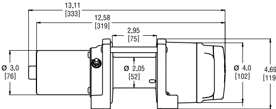
Winch dimensions: 13.1” L. x 4.53” D. x 4.69” H. (33.3Cm L. x 11.5Cm D. x 11.9Cm H.)
